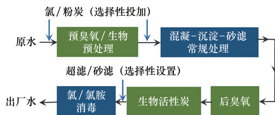
图2 长三角地区典型饮用水处理工艺流程
