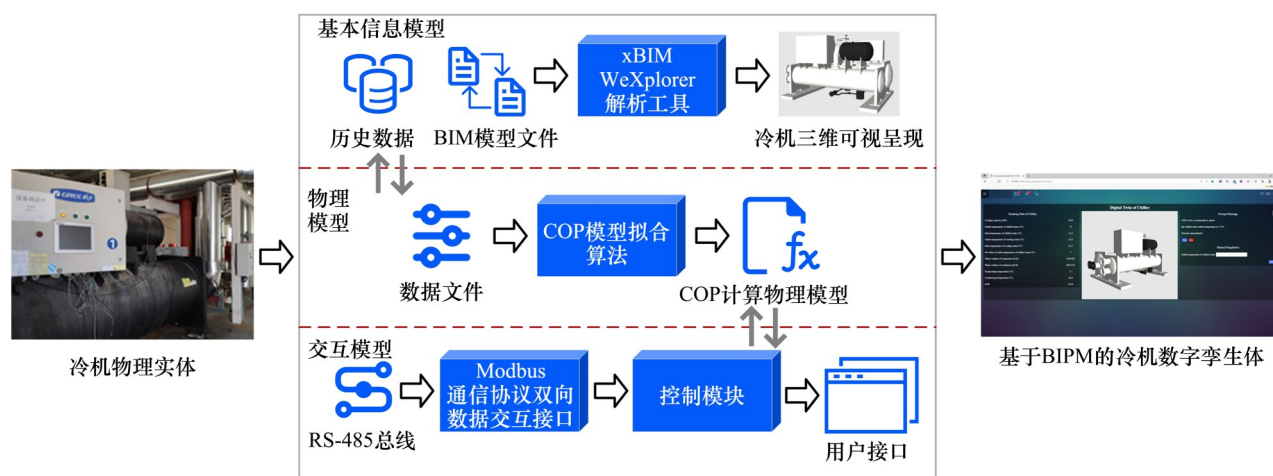
图4 基于BIPM的冷机数字孪生系统实现原理
