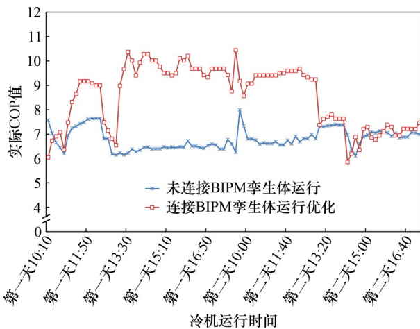
图 5 物理冷机连接 BIPM 孪生体前后运行 COP 结果对比 注：横坐标时刻非均匀放置。
