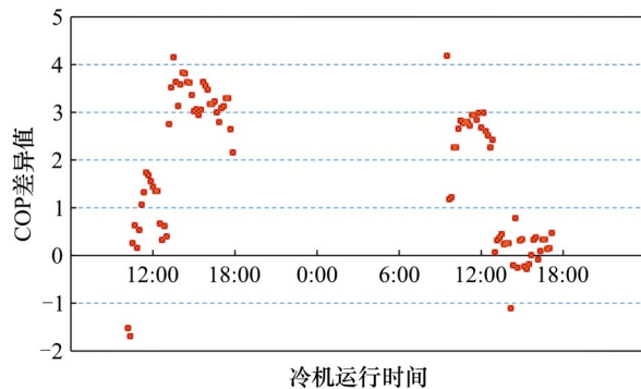
图 6 物理冷机连接 BIPM 孪生体前后运行 COP 差异值对比
