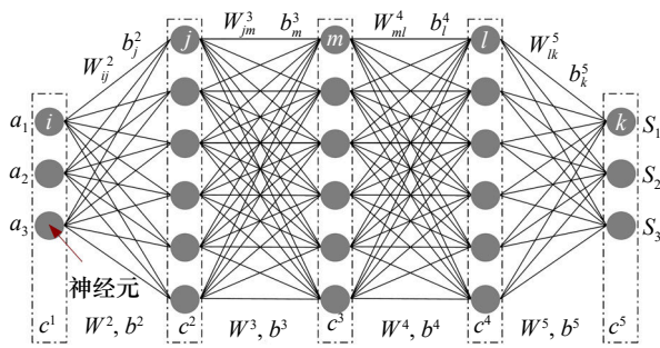
图1 基于神经网络算法训练等效本构关系示意图
