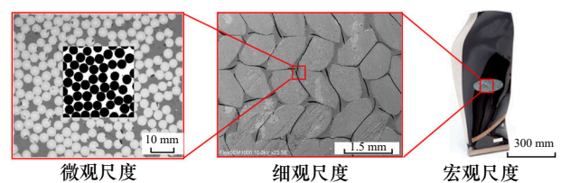
图3 编织复合材料不同尺度结构示意图
