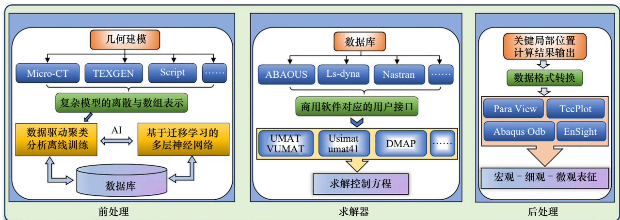
图4 先进复合材料结构一体化多尺度计算平台示意图
