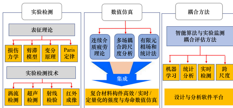
图5 复合材料构件强度与寿命仿真评价方法体系
