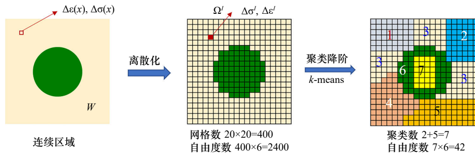
图2 数据驱动自洽聚类分析仿真方法示意图
