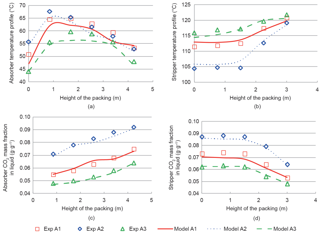
图7. 模型预测和实验数据的验证结果：(a) 吸收塔温度分布；(b) 汽提塔温度分布；(c) 吸收塔 CO_2 浓度分布；(d) 汽提塔 CO_2 浓度分布。Exp: 实验数据；Model: 模型预测。
