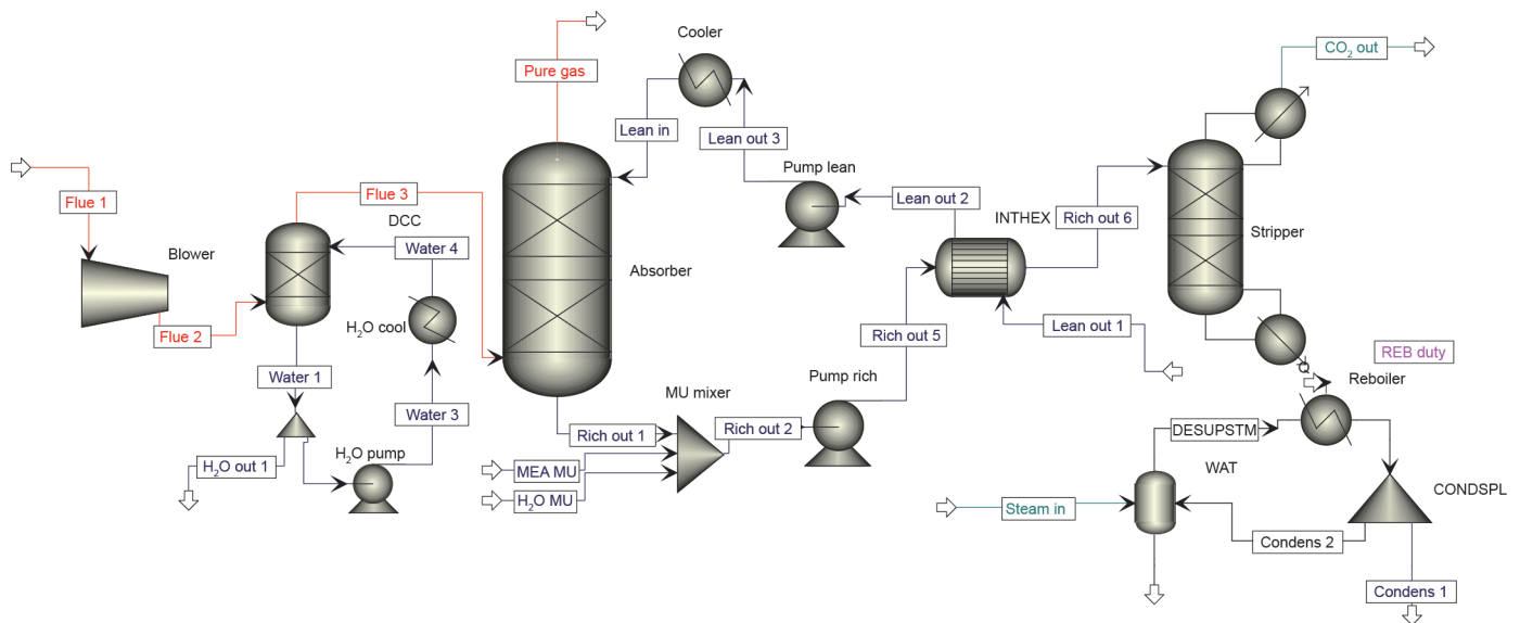
图5. Aspen Plus®工艺流程图。MU: 补充; REB:再沸器; CONDSPL: 凝液分离器; DESUPSTM: 不饱和蒸汽; INTHEX: 中间换热器; DCC: 直接接触冷却塔; WAT: 水蒸气降温器。
