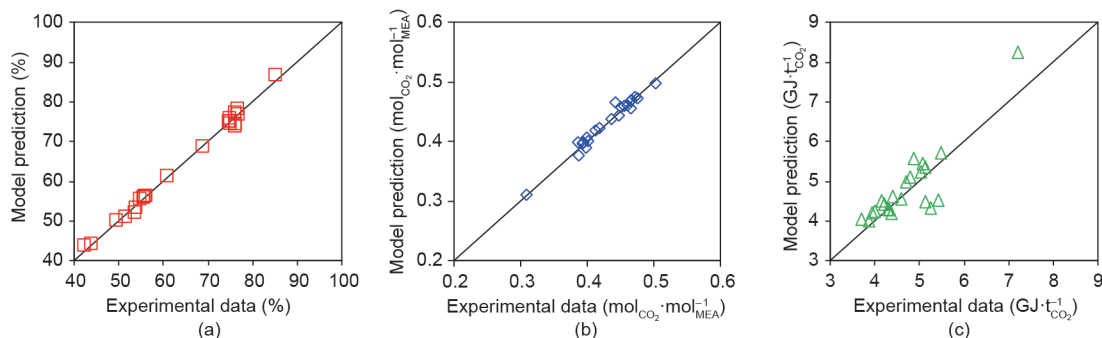
图6. 模型预测和实验数据的偏差: (a) \text{CO}_2 捕集率; (b) 富溶剂中 \text{CO}_2 载荷; (c) \text{CO}_2 特征热负荷。
