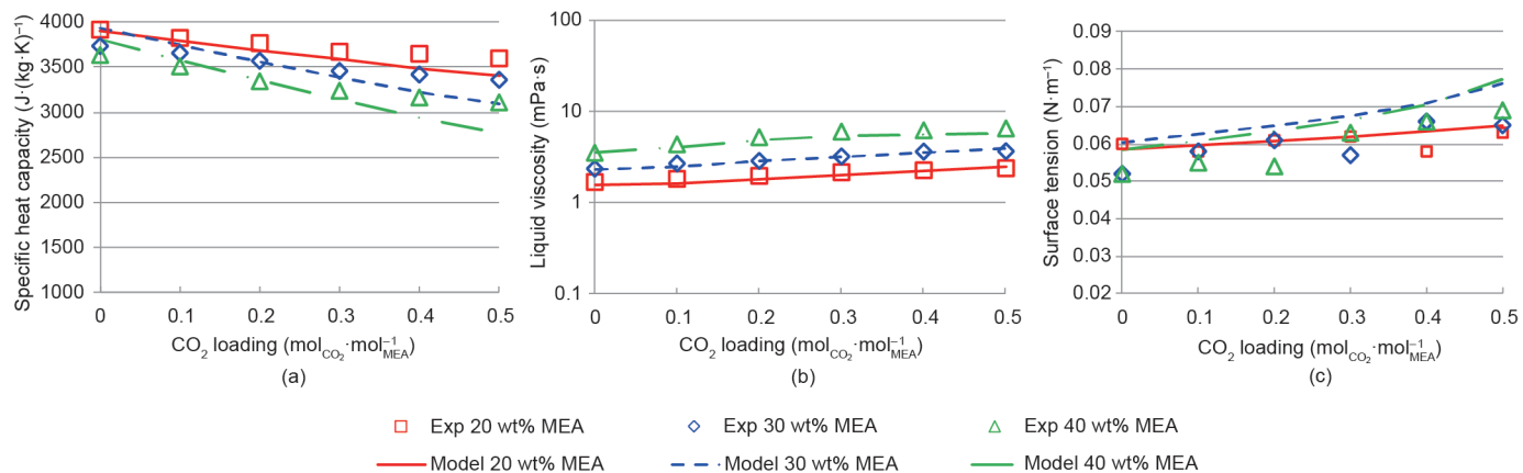
图4. 298.15 K温度下MEA-H 2 O-CO 2 物系的物性计算验证结果: (a) 液相热容; (b) 液相黏度; (c) 液相表面张力。Exp: 实验数据; Model: 模型预测。
