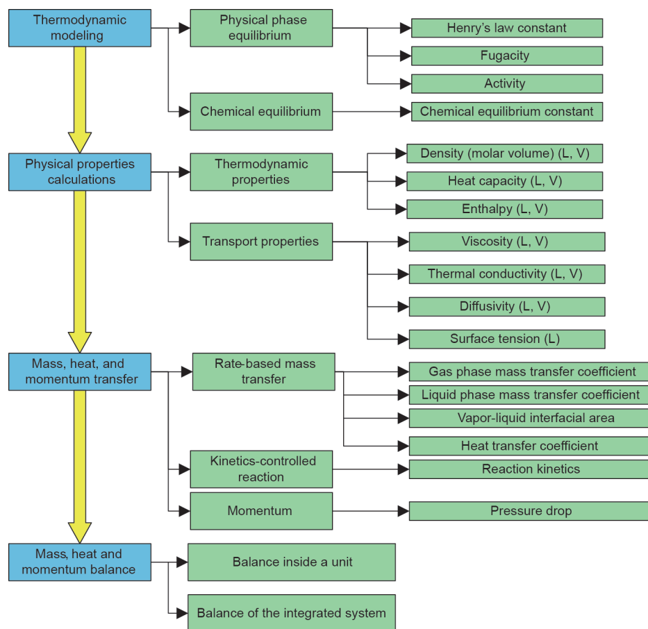
图1. PCC工艺碳捕集过程模型框架示意图。L: 液相; V: 气相。
