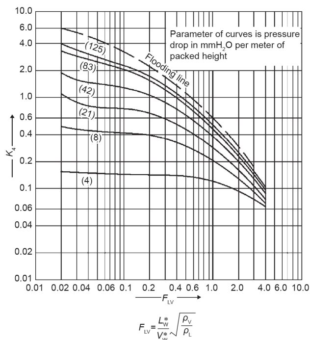
图8. 通用压降关联图[64]。
