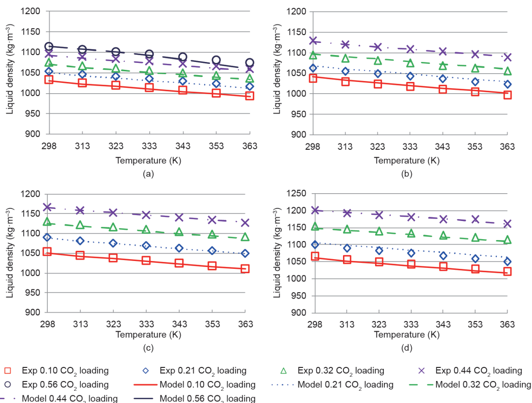
图3. MEA-H 2 O-CO 2 物系的液相密度计算验证结果: (a) 30 wt% MEA溶剂; (b) 40 wt% MEA溶剂; (c) 50 wt% MEA溶剂; (d) 60 wt% MEA溶剂。Exp: 实验数据; Model: 模型预测。
