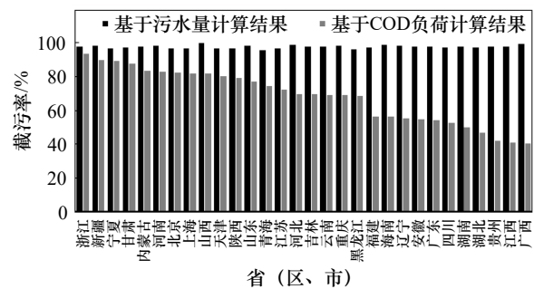
图3 30个省（区、市）的统计污水收集率和实际污水收集率对比
