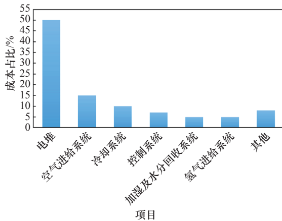
(b) 燃料电池系统成本构成
