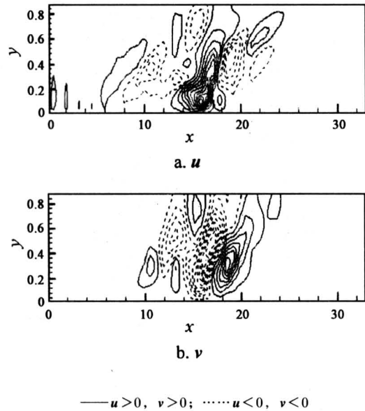
图2 扰动速度 u, v 在 x - y 平面上的分布
