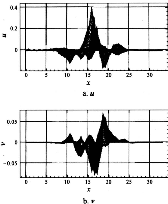
图1 扰动速度 u, v 的三维分布
