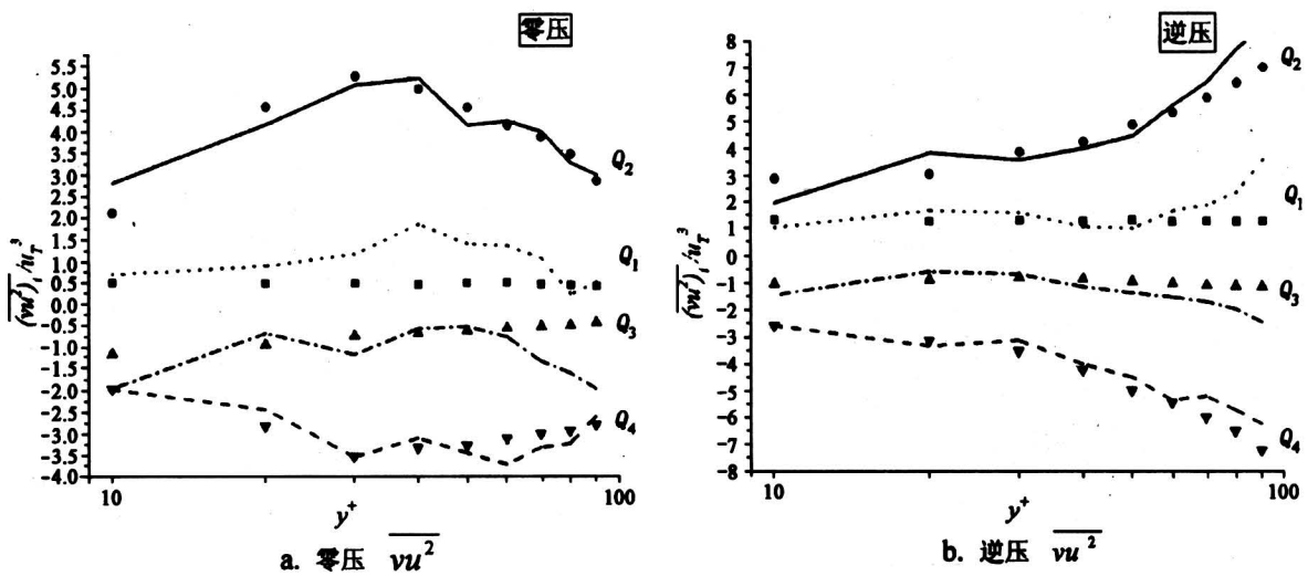
图5 零压、逆压下 Q_1, Q_2, Q_3, Q_4 对 \overline{vu^2} 的贡献
