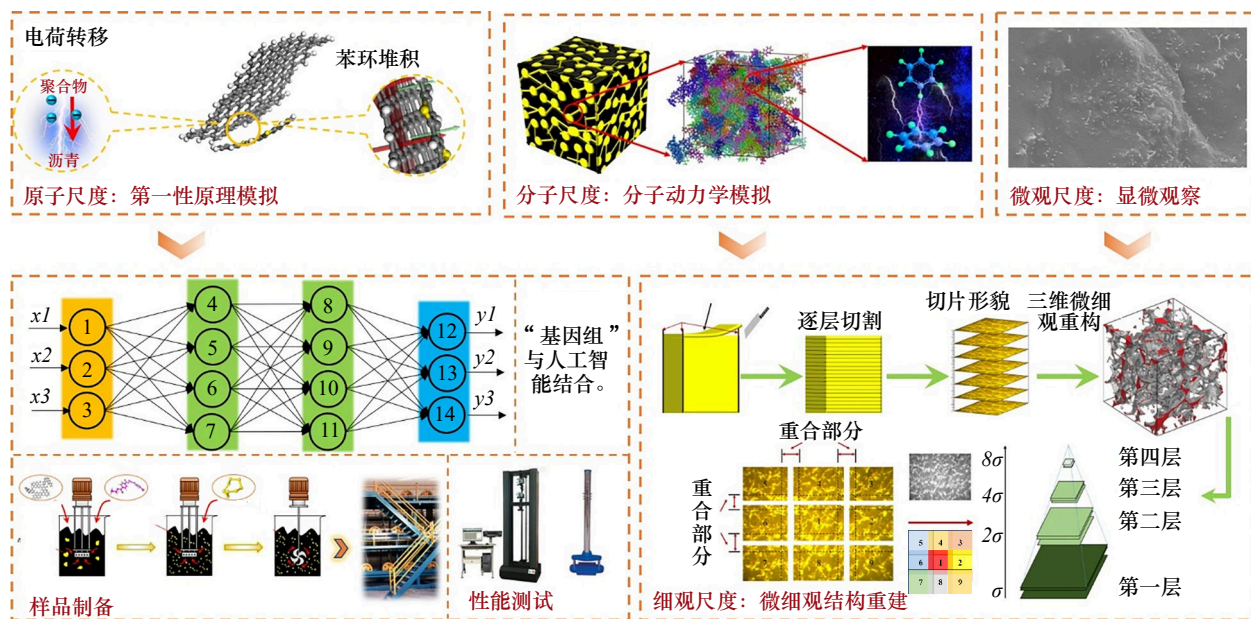
图2 防水卷材多尺度性能评估技术路线
