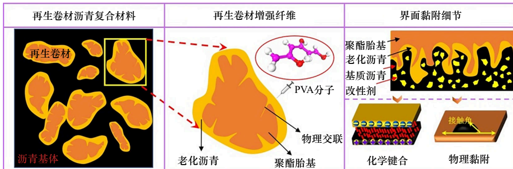
图5 废弃沥青基防水卷材界面多尺度作用
