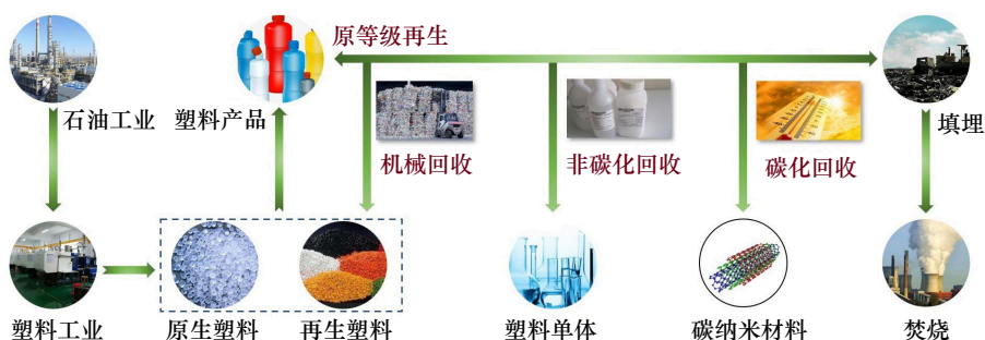
图3 废弃高分子材料（以塑料为例）的多级再生策略
