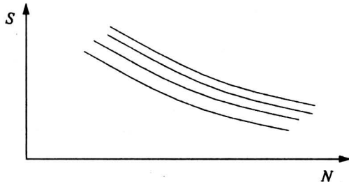
图 2 动态的 S-N 曲线
