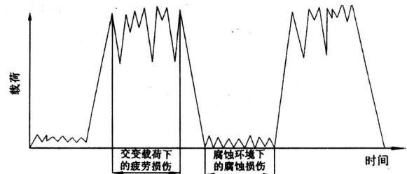
图 1 飞机结构的载荷 - 环境 - 时间历程示意
