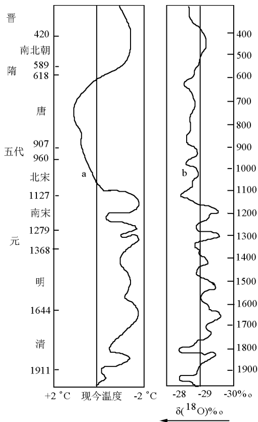
a—依据中国物候资料；b—依据格陵兰冰雪资料 同位素测量 \delta(^{18}\text{O}) 每增加 0.69\text{‰} 温度升高 1^\circ\text{C}
