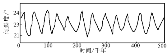
图3 50 万年间地球轨道及旋转轴倾斜角度变化
