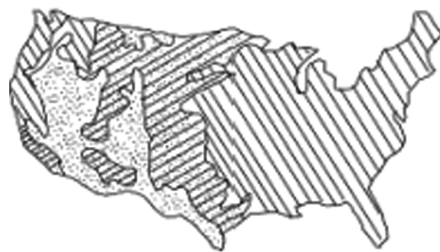
(b) 1915年干旱区缩减图
