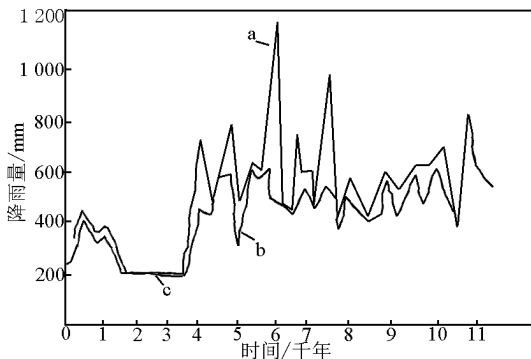
a—年平均；b—夏季风期；c—干旱期
