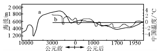
图中1600 m处为目前挪威雪线高度,0作为目前温度 横线时间比例尺是幂数的,越向左越小。 a—挪威雪线高度;b—中国温度
