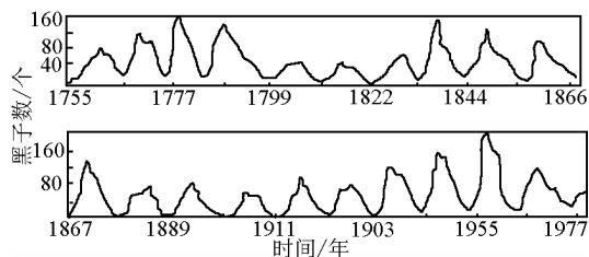
图4 220 年来太阳黑子数变化图
