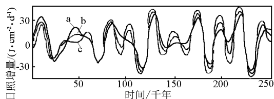
a—65° N; b—55° N; c—45° N
