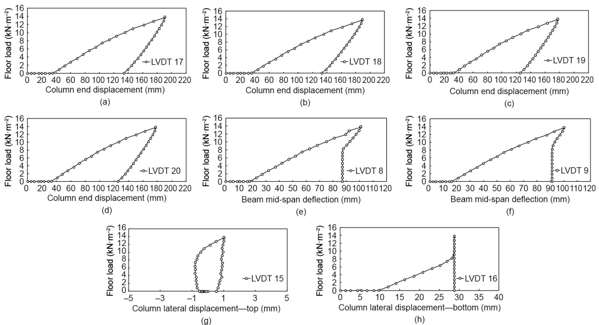
Fig. 21. Measured displacements: (a) LVDT 17; (b) LVDT 18; (c) LVDT 19; (d) LVDT 20; (e) LVDT 8; (f) LVDT 9; (g) LVDT 15; (h) LVDT 16.
