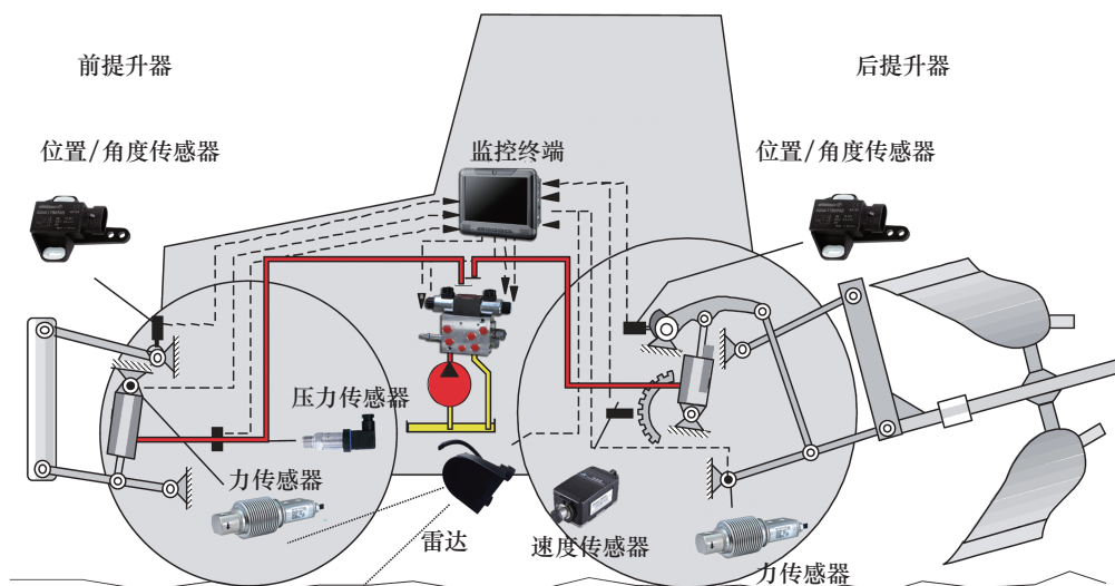
图1 耕整地机械耕深控制系统示意图
